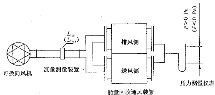
图 C.1 外部漏风率测量装置
